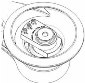
1. Einstellung der Maschine bei Auslieferung. 2. Einstellung der Maschine mit Schutz- oder Softauflage.
